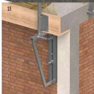
Bekistingsbalk
