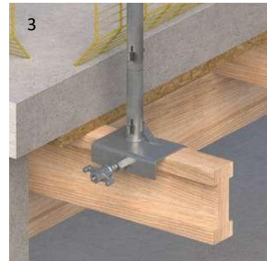
Balkbevestiging
