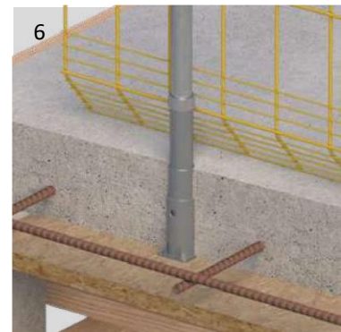
Horizontale instorthuls
