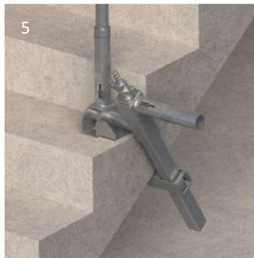
Trap bevestiging
